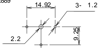
取付穴参考寸法 (スイッチ搭載面)
